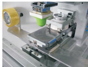
Kretanje platforme napred/nazad
